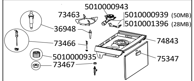
Jets / Injecteurs 28mb 5010002448 Model 2-3-4 Classic L Deluxe
