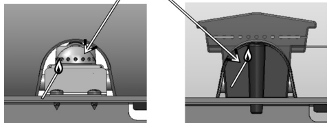
καυστήρας από ανοξείδωτο ασάλι καυστήρας από χυτοσίδηρο
