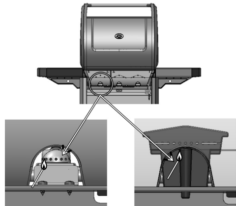
roestvrijstalen brander
