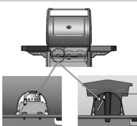
horák z nehrdzavejúcej ocele
