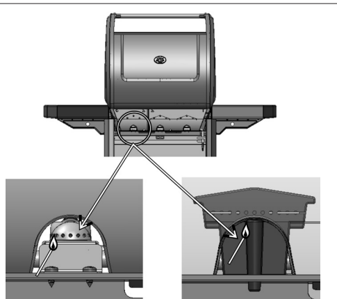
gorilnik iz nerjavnega jekla
