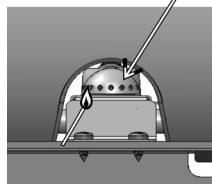
rozsdamentes gázégő
