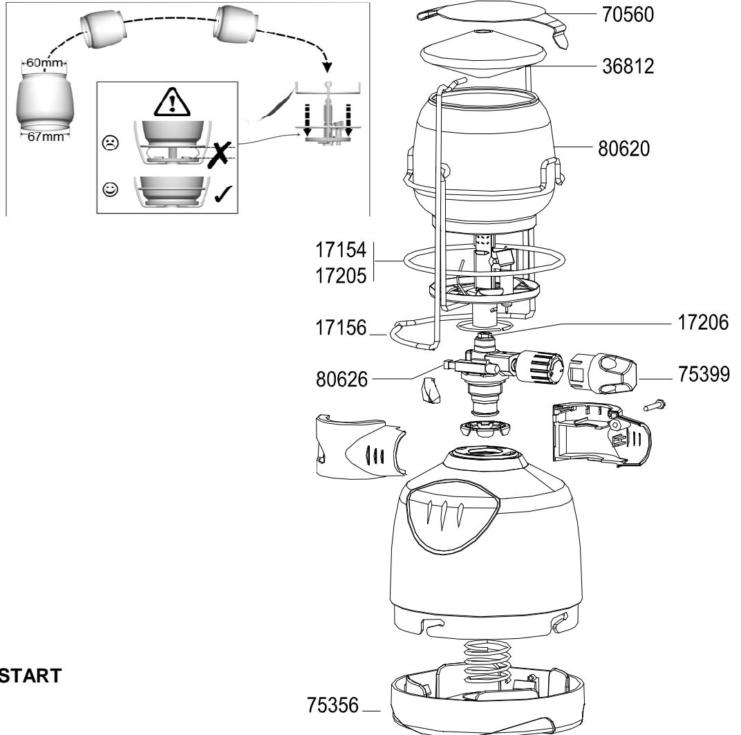
BLEUET CV 300 L
